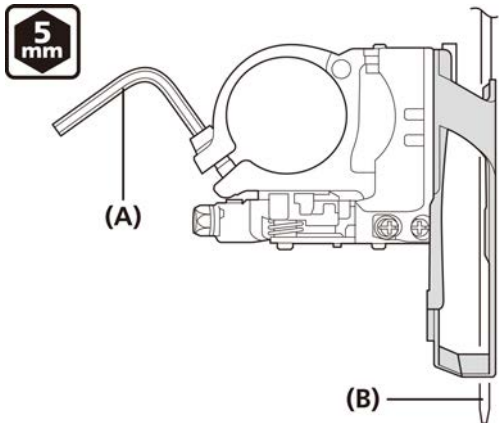
(A) Шестигранный ключ на 5 мм (B) Наибольшая передняя звезда
