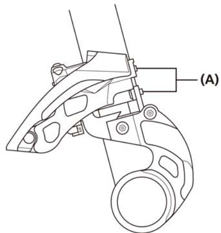
(A) Линк
