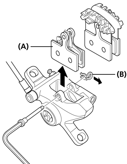
(A) Тормозная колодка (B) Пружинное запорное кольцо
