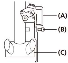
(A) Передний переключатель (B) Болт (C) Положение каретки
