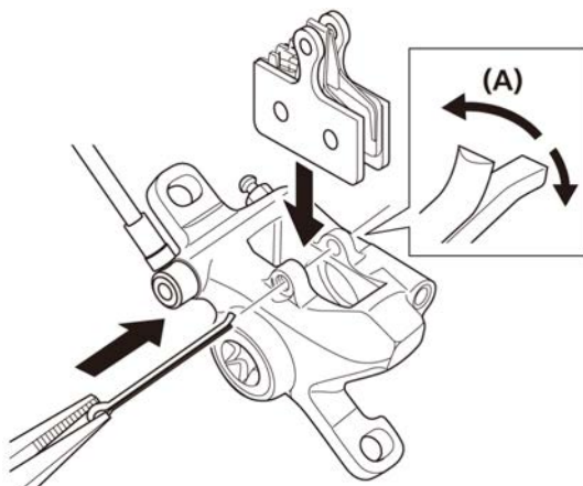
(A) Шплинт
