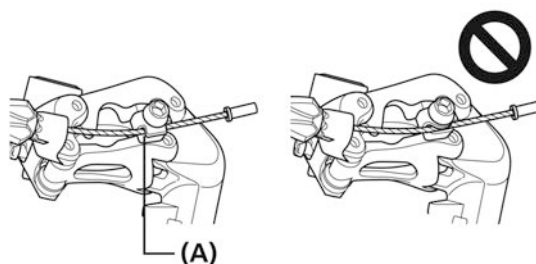
(A) Канавка
